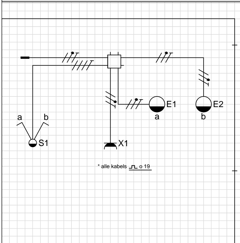
Installatieschema
